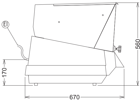
Oldalnézet
